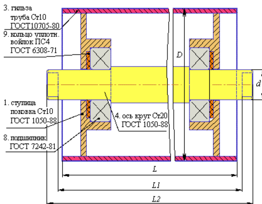
Ролик конвейерный неразборный: составные части и основные размеры
