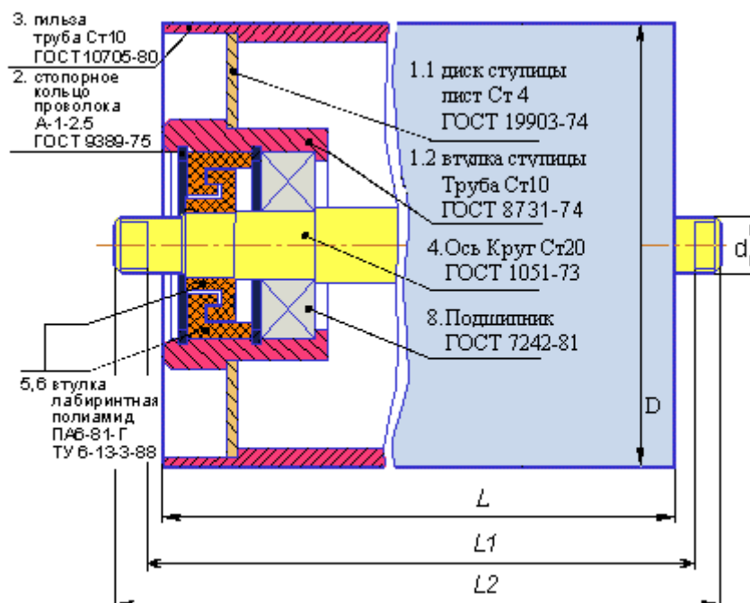
Ролик конвейерный разборный: составные части и основные размеры
